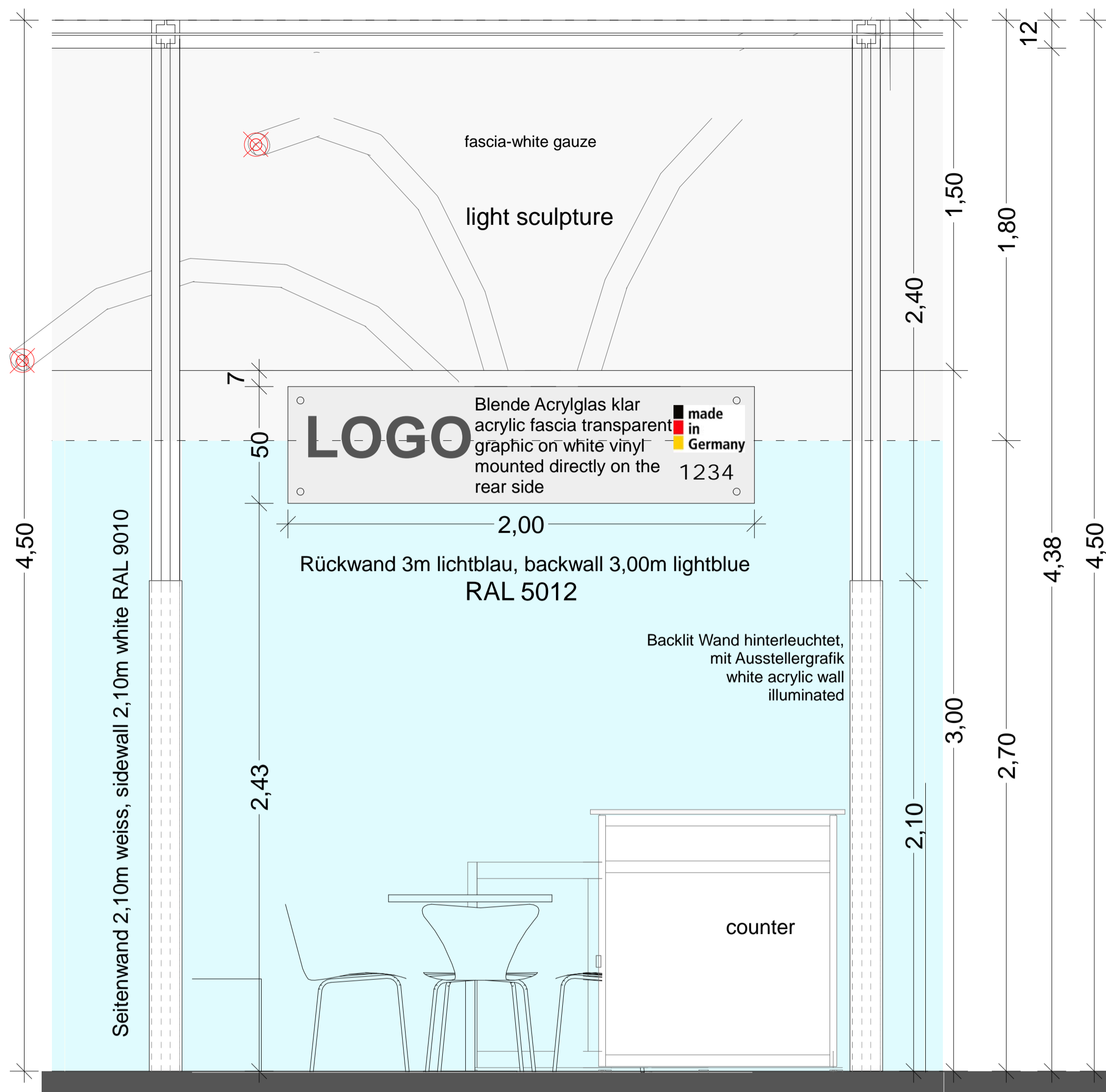
Vorderansicht/ front view
