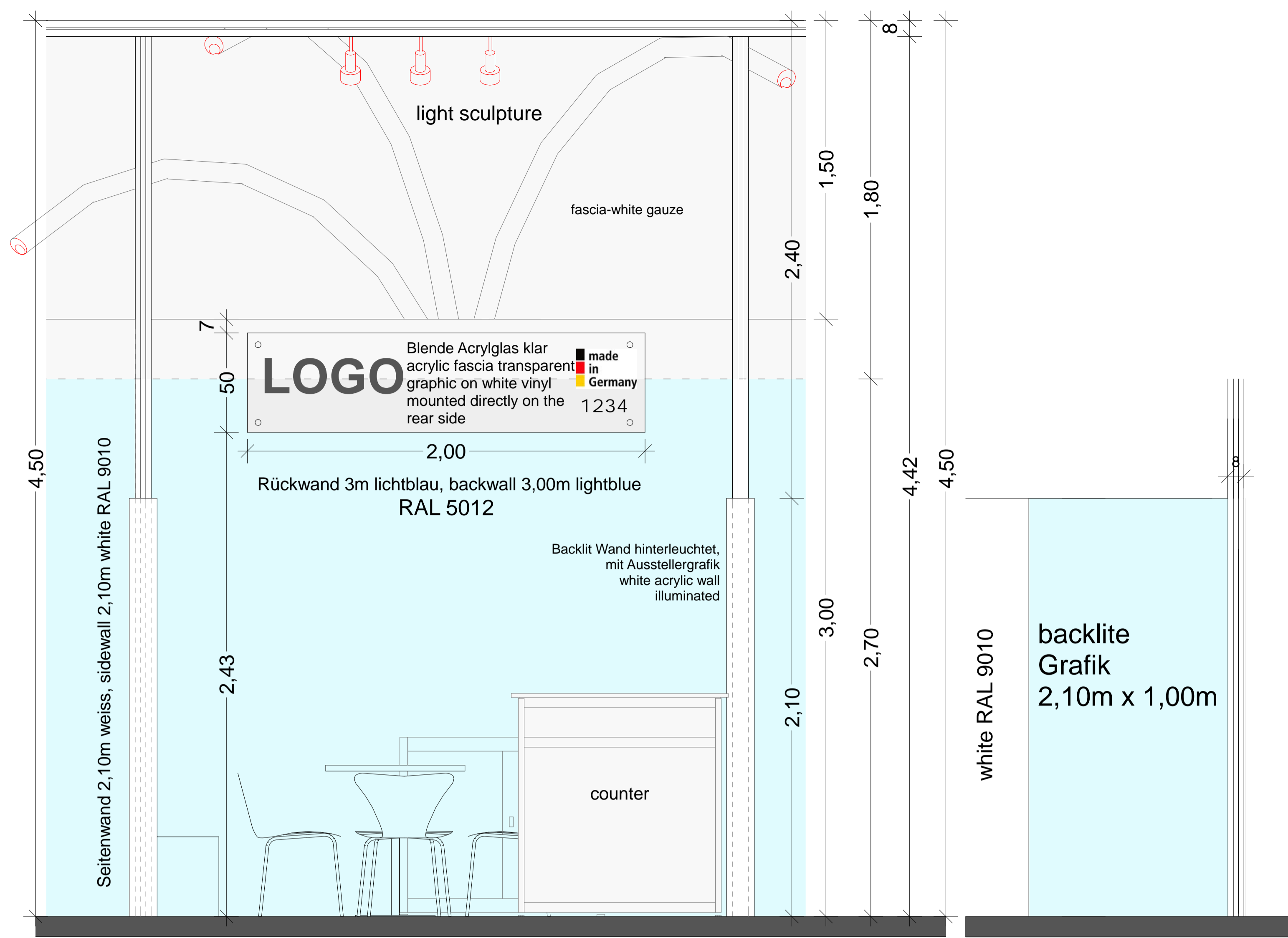
Vorderansicht/ front view
