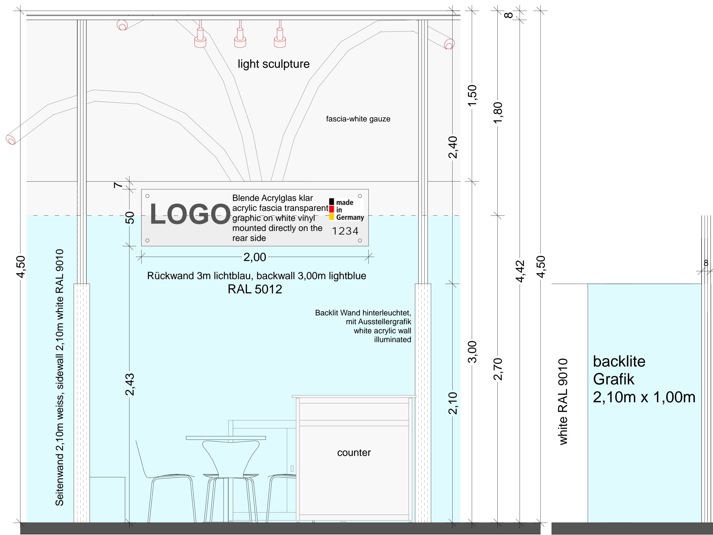
Vorderansicht/ front view
