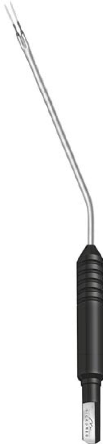
127-122-110 110 mm Elektrode HNO, 30° gebogen, Spitze 45° gebogen Électrode ENT, 30° curved, tip 45° curved Électrode ORL, coudée 30°, pointe coudée 45° Electrodo otorrino, curvo 30°, punta curvo 45° Elettrodo otorino, ricurvo 30°, punta ricurvo 45°
