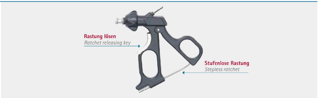
128-100-081 Ergonomischer Handgriff mit stufenloser Rastung, Rastung lösendem Modul und HF-Verbindung Ergonomic highly rigid ring handle with stepless ratchet, ratchet releasing key, rotation module and HF connection
